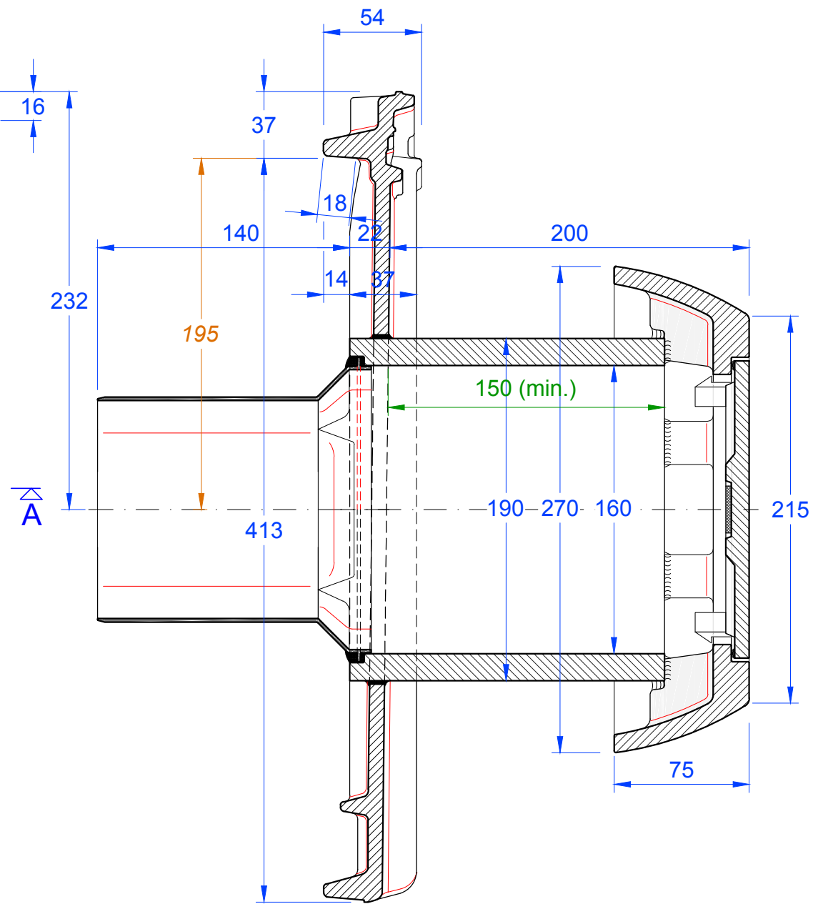
Schnitt B-B
