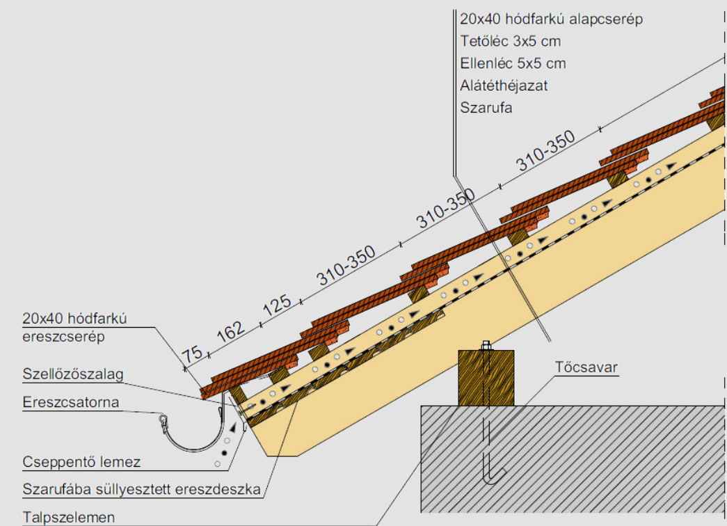
Koronafedésű ereszkialakítás
