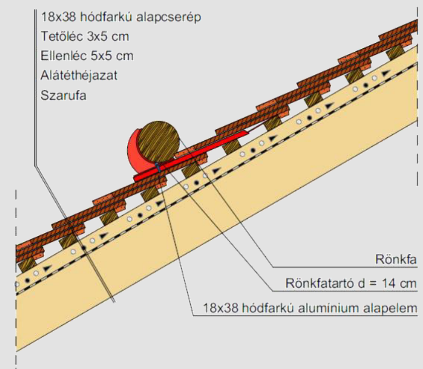
Rönkfatartó elhelyezése
