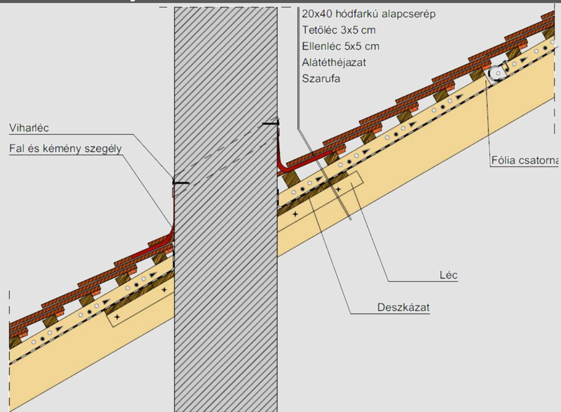
Kéményszegély kialakítás
