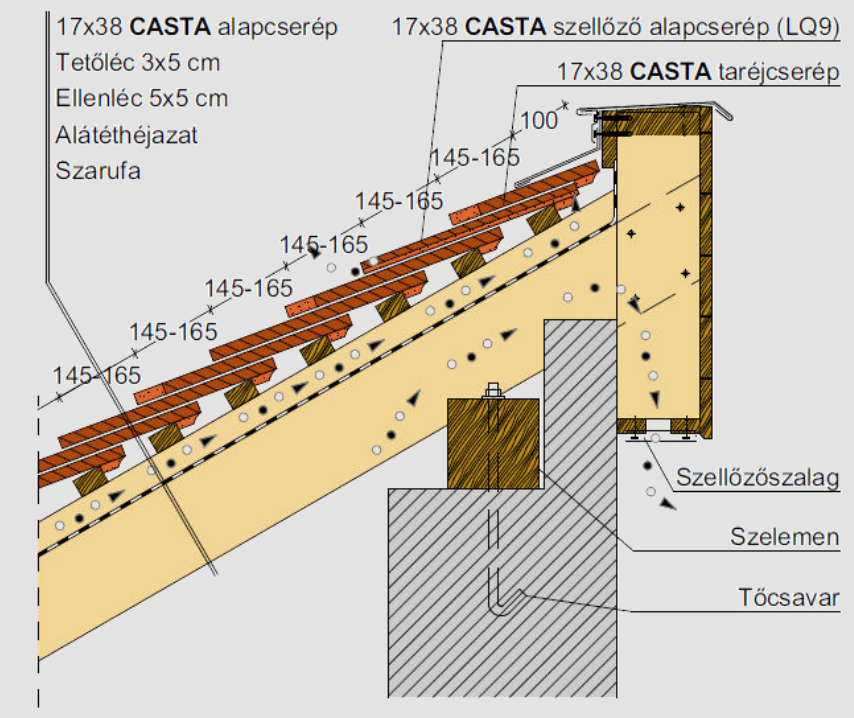
Félnyeregűtető gerinc kialakítás
