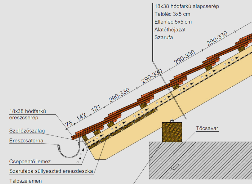
Koronafedésű ereszkialakítás
