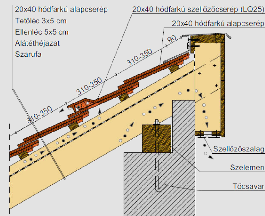
Koronafedésű félnyeregtes gerinc kialakítás
