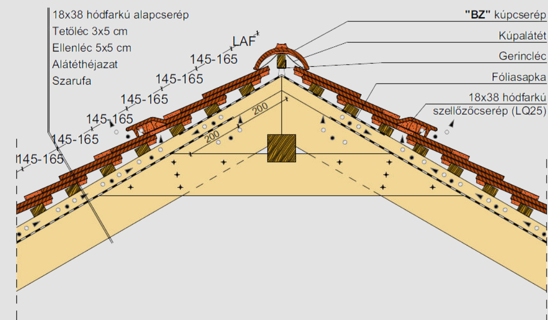
Gerinckialakítás, szellőzőcseréppel
