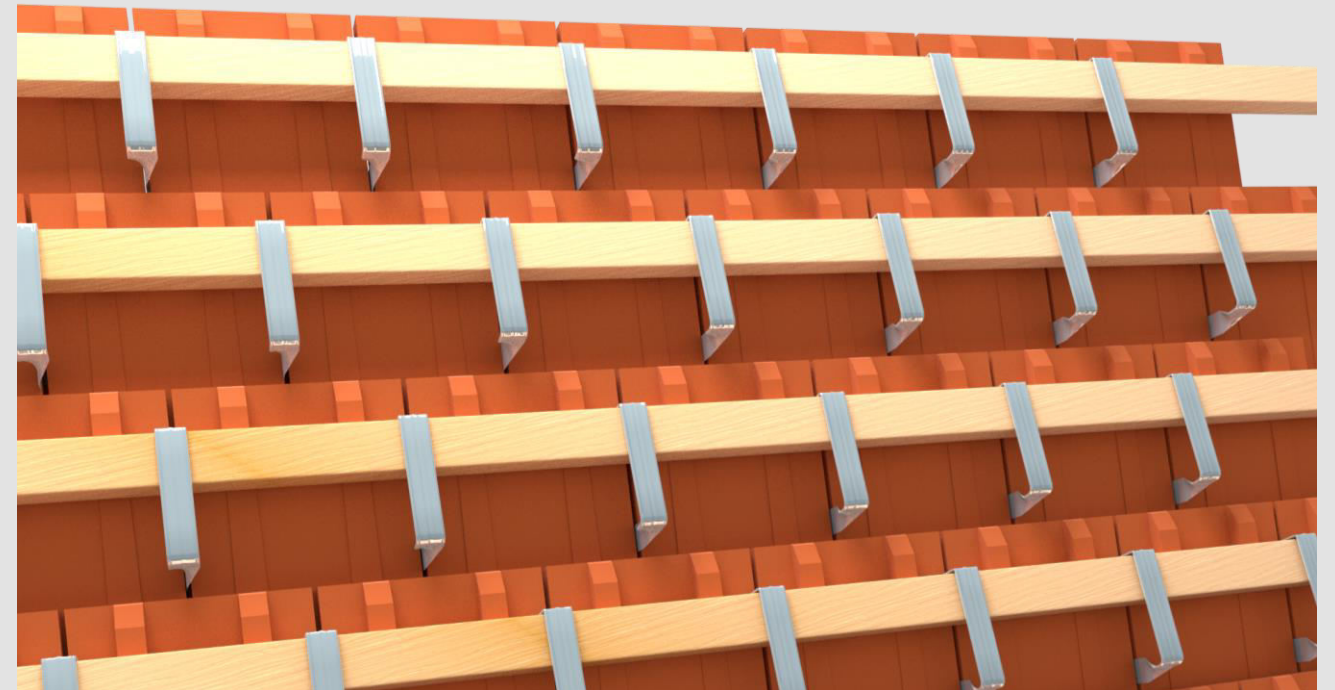
Séma 1:1 beakasztós viharkapocshoz, kettősfedésű hódfarkú cserépfedéshez
