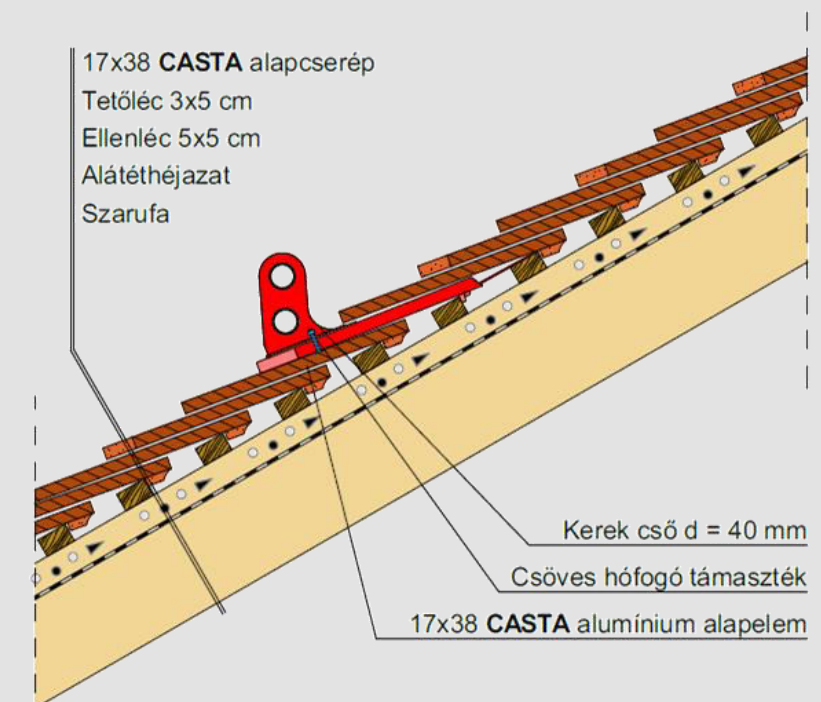
Hófogócső elhelyezése
