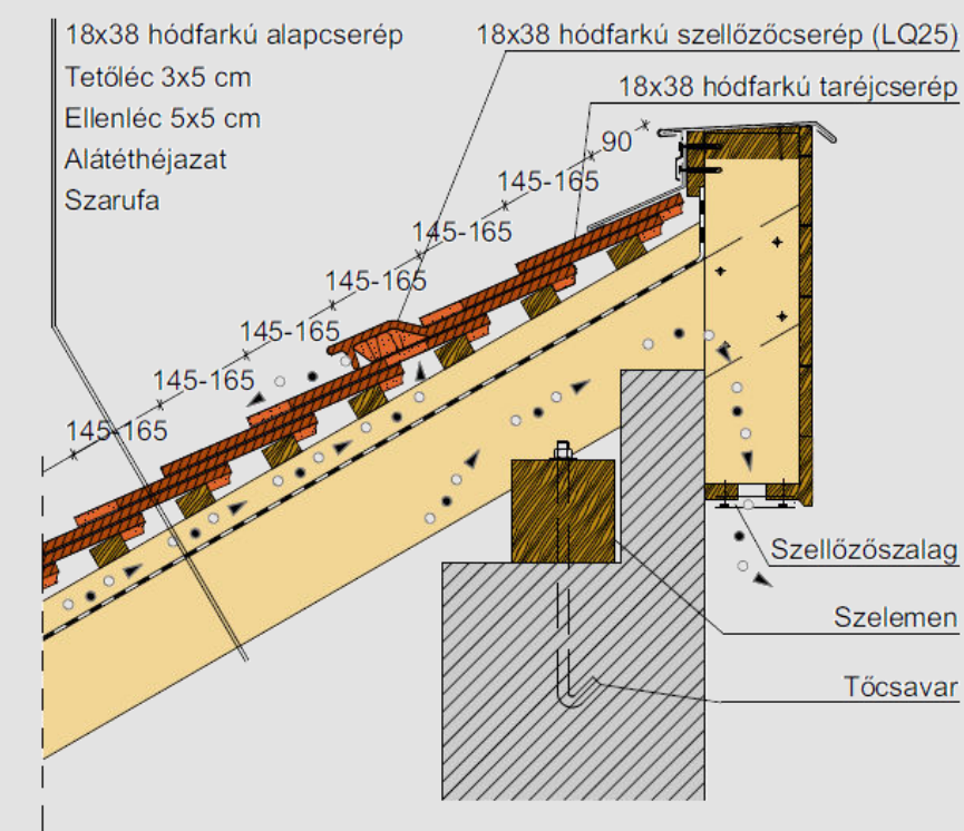
Félnyeregű gerinc kialakítás
