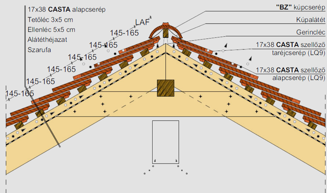
Gerinckialakítás, szellőző alapcseréppel és szellőző taréjcsereppel
