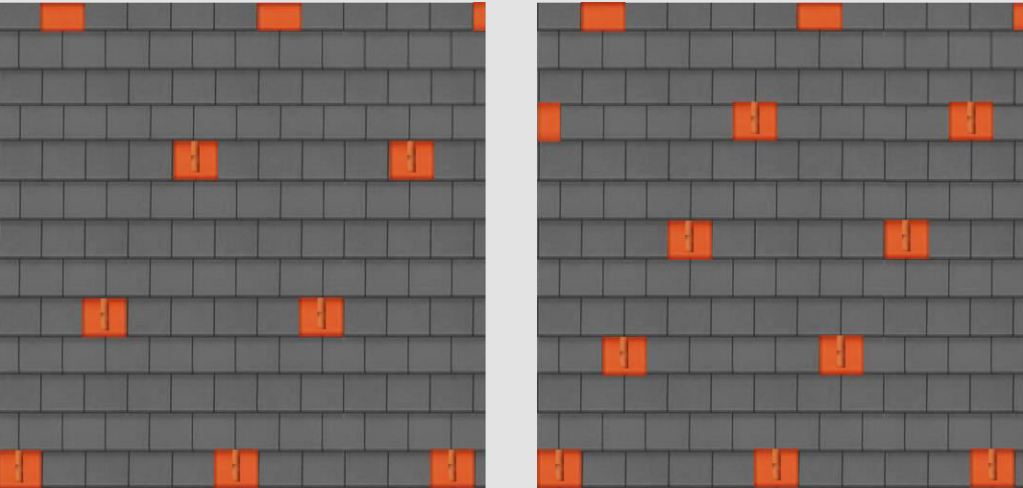
CREATON "Bécsi táska", kettősfedésben, 33,3 db/m 2 anyagigénnyel
