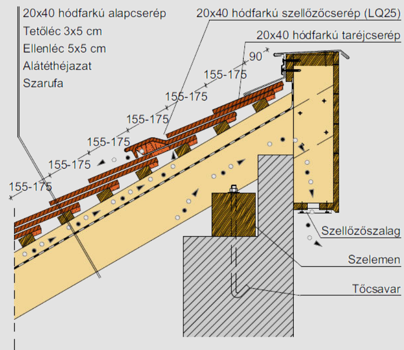
Félnyereg tető gerinc kialakítás
