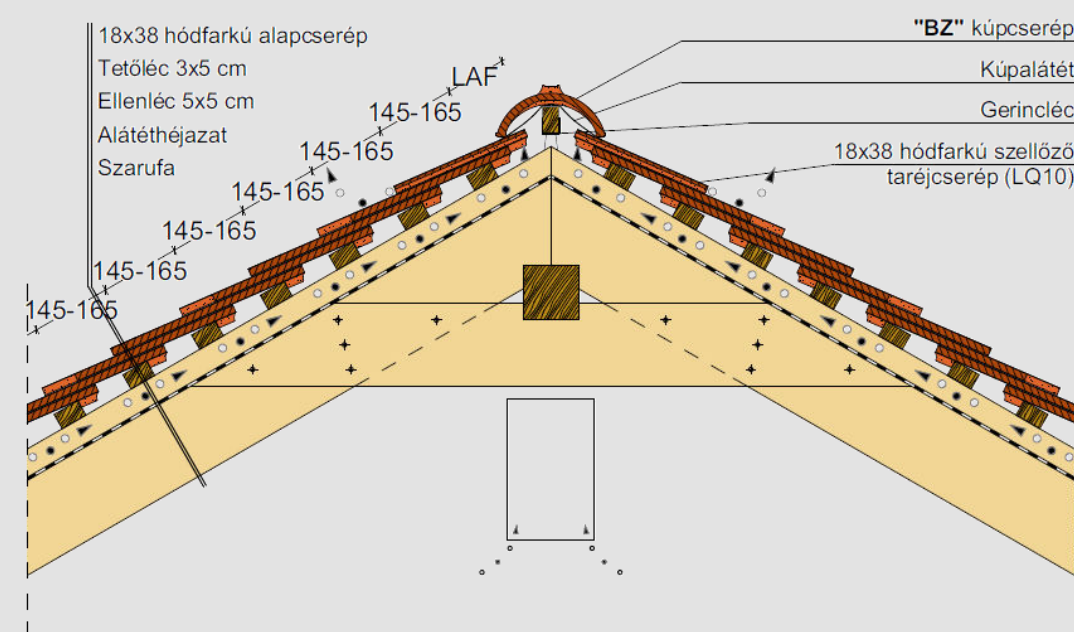
Gerinckialakítás, szellőző taréjcsereppel
