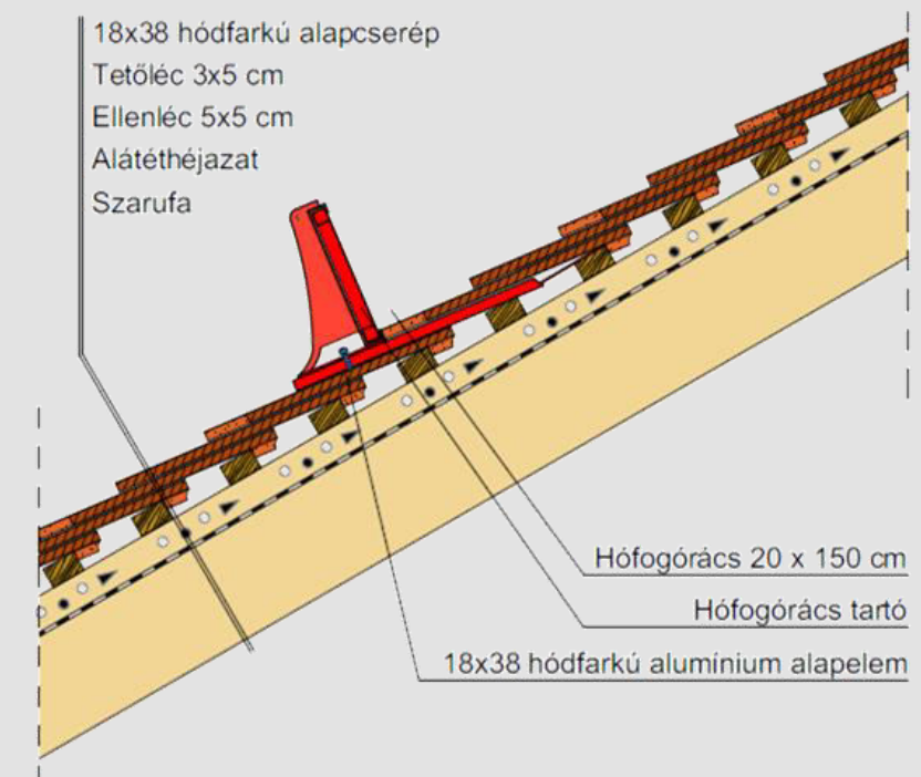
Hófogórács elhelyezése
