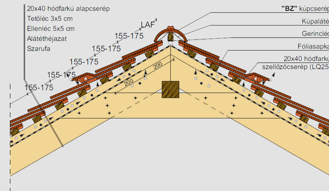
Gerinckialakítás, szellőzőcseréppel
