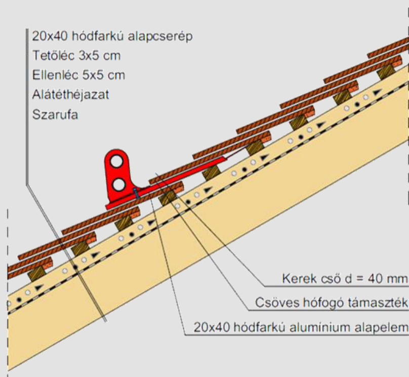
Hófogócső elhelyezése
