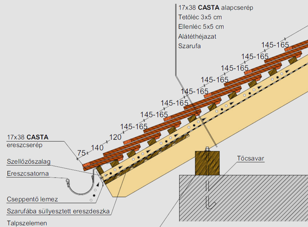
Ereszkialakítás
