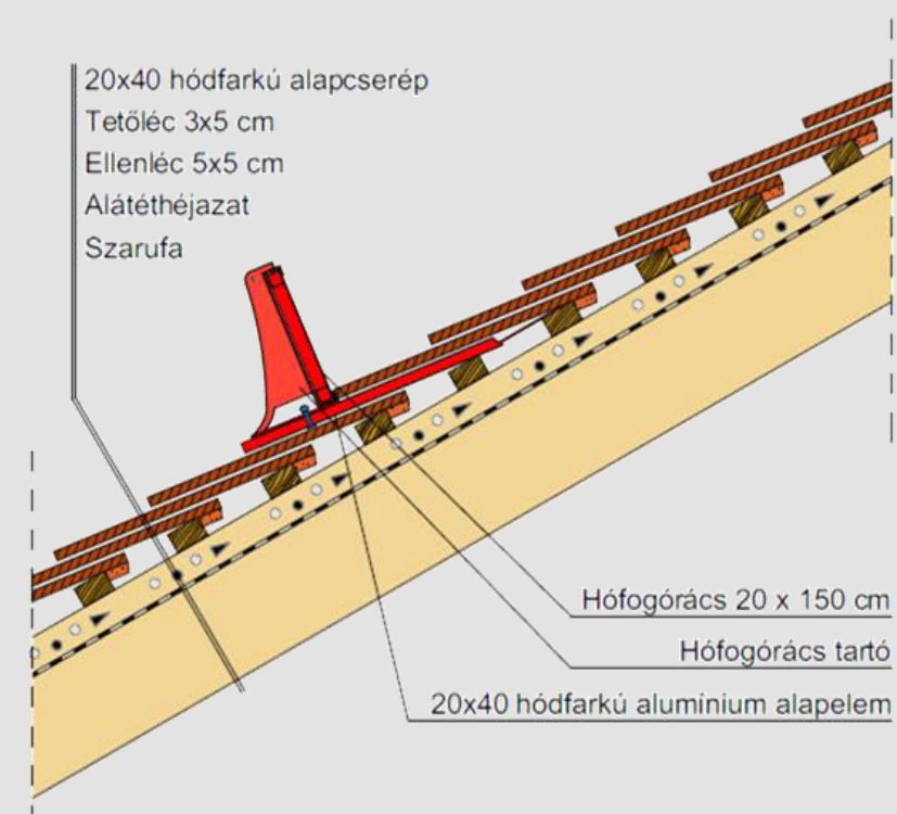
Hófogórács elhelyezése
