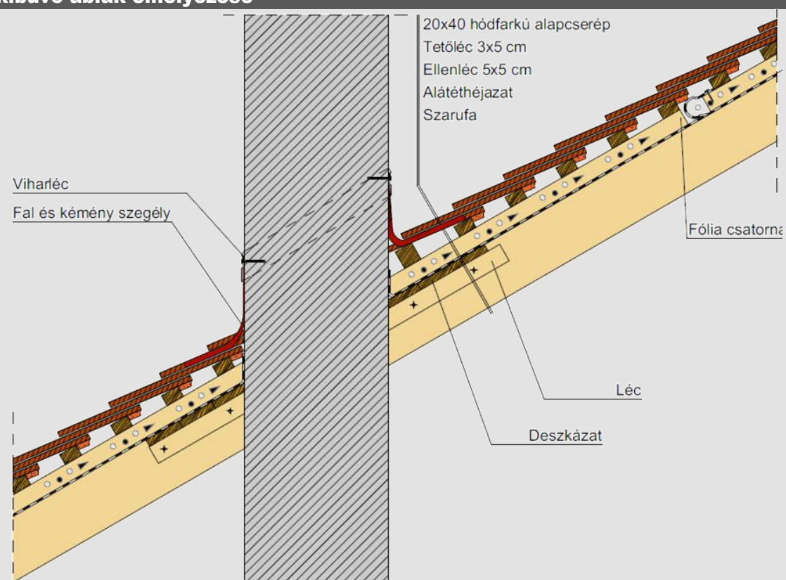
Kéményszegély kialakítás
