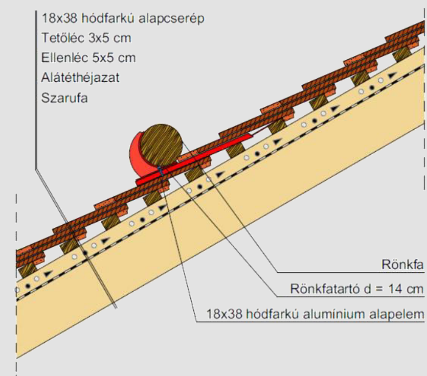
Rönkfatartó elhelyezése
