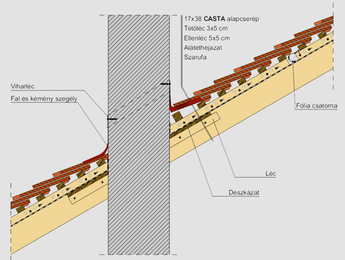
Kéményszegély kialakítás
