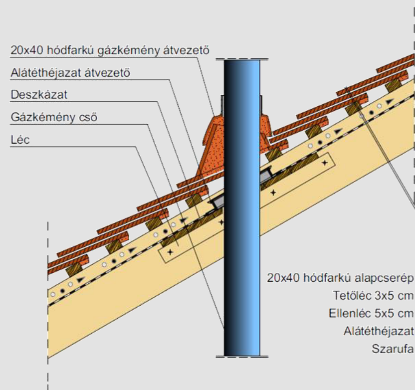
Kerámia gázkémény átvezető rendszer
