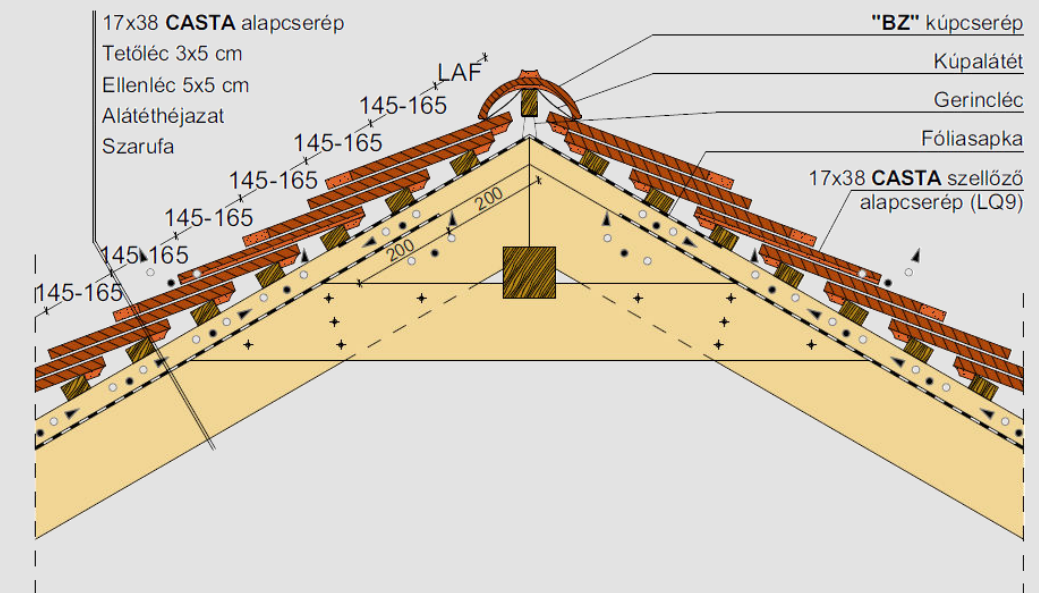
Gerinckialakítás, fóliasapkával
