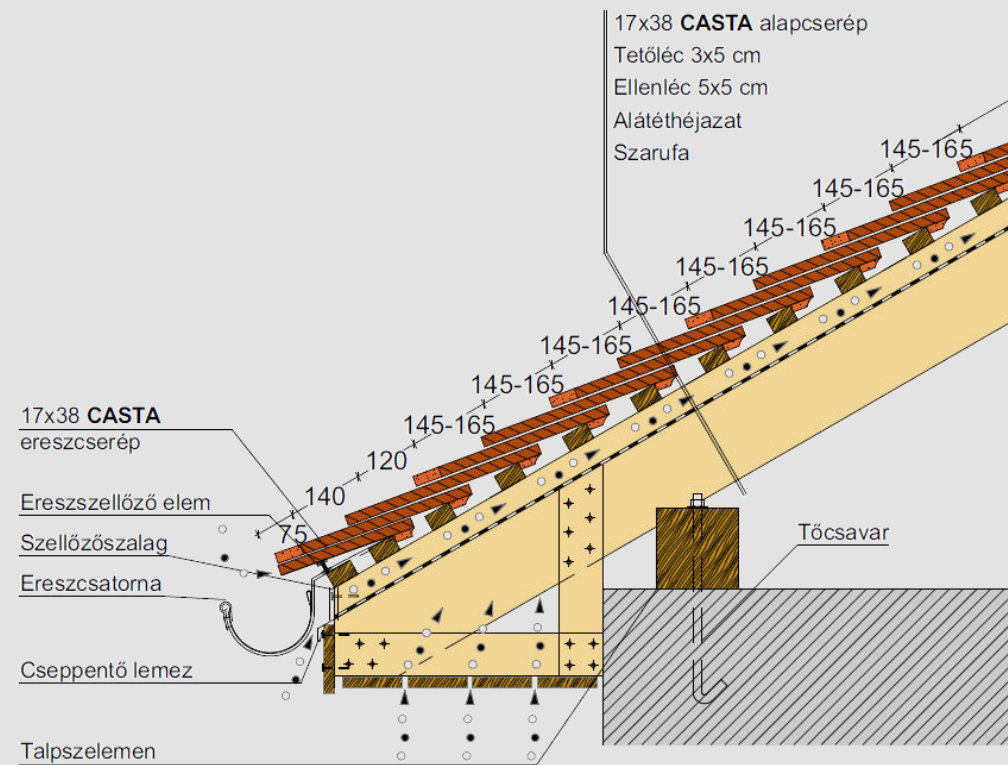
Dobozolt ereszkialakítás
