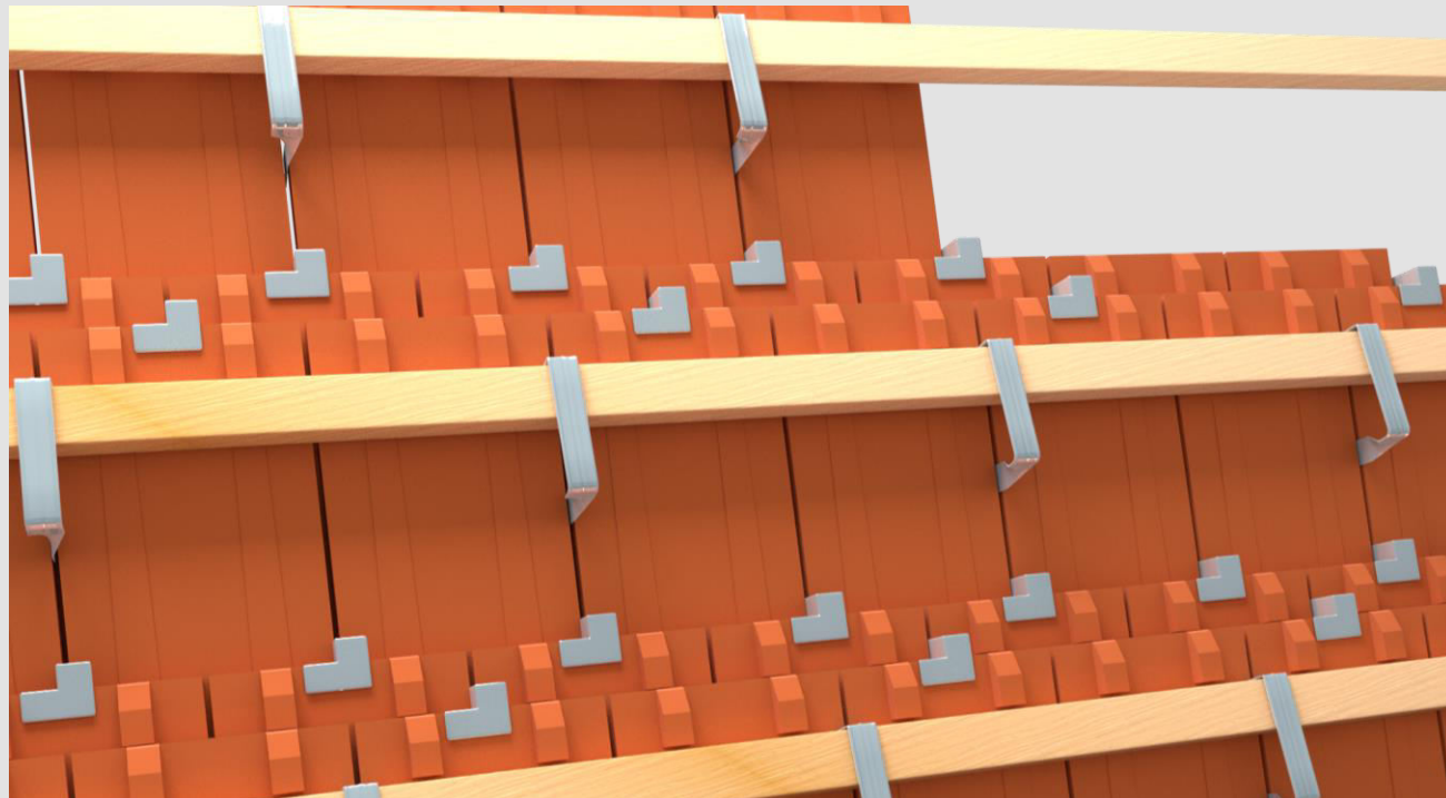
Séma a beakasztós viharkapocs használatához, koronafedésű hódfarkú cserépfedéshez
