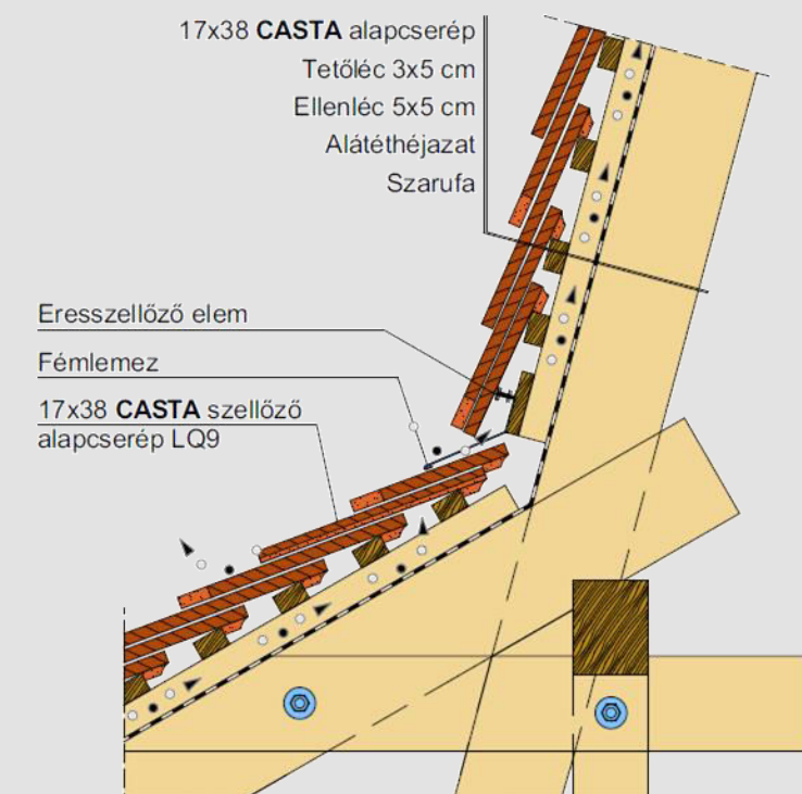
Pozitív hajlásszögűtörés kialakítás
