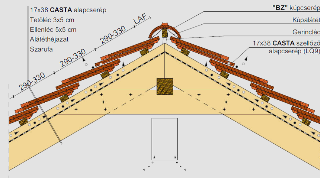
Koronafedésű gerinckialakítás, szellőző alapcseréppel
