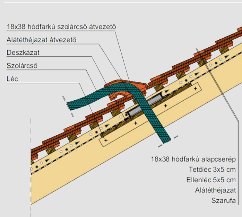
Kerámia szolár cső átvezető rendszer
