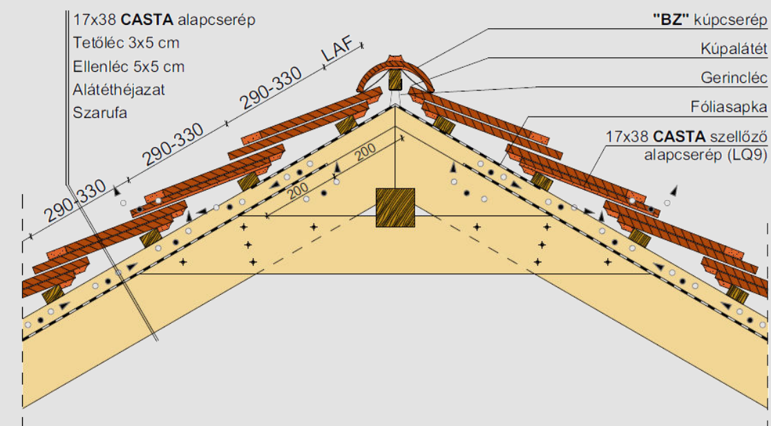
Koronafedésű gerinckialakítás, szellőzőcseréppel,
