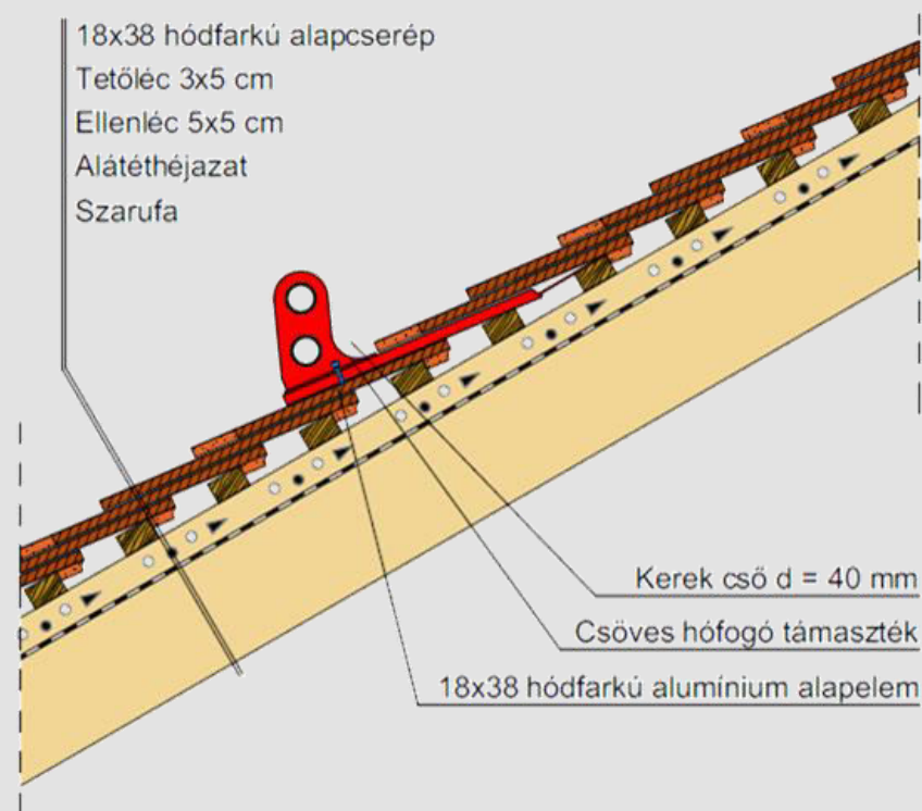
Hófogócső elhelyezése
