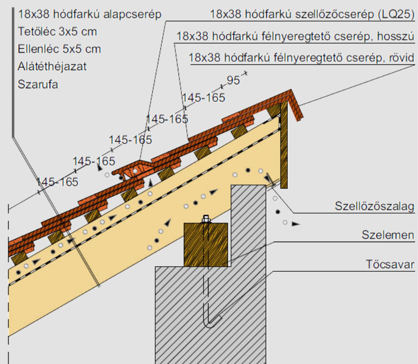
Félnyeregvető gerinc kialakítás, félnyeregvető cseréppel
