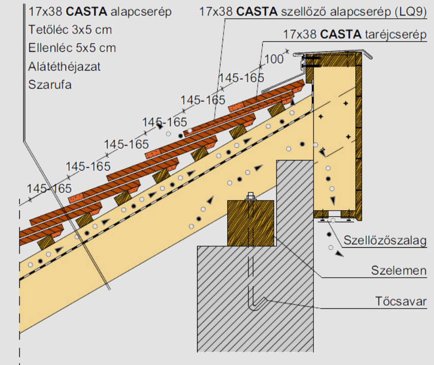
Félnyeregű gerinc kialakítás
