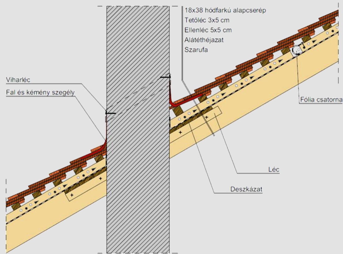
Kéményszegély kialakítás
