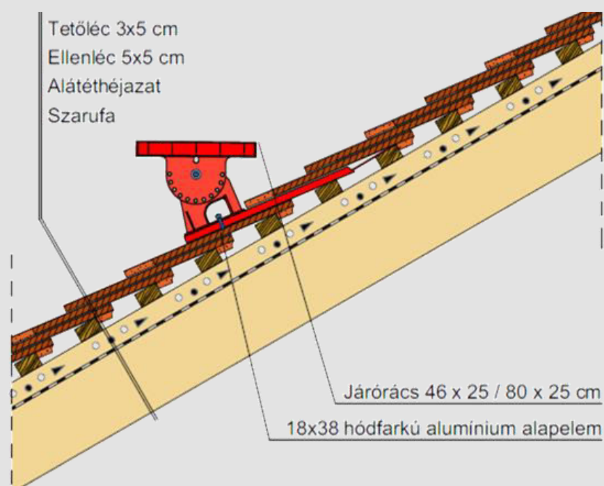
Járórács elhelyezése
