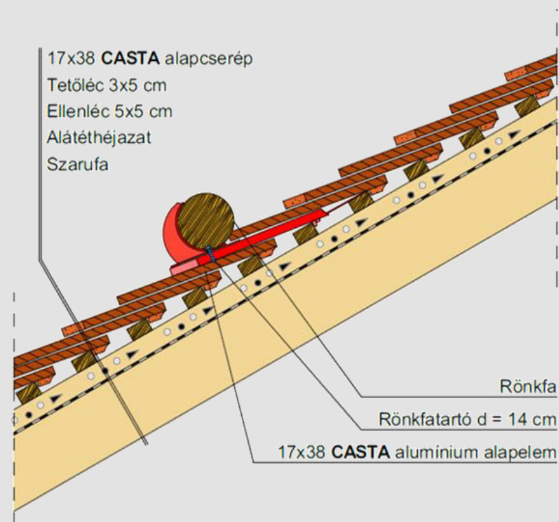
Rönkfartó elhelyezése
