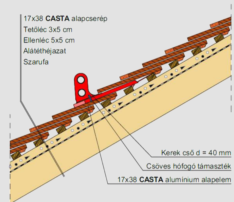
Hófogócső elhelyezése
