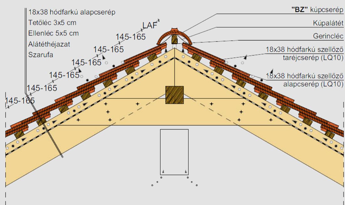
Gerinckialakítás, szellőző taréj- és szellőző alapcseréppel
