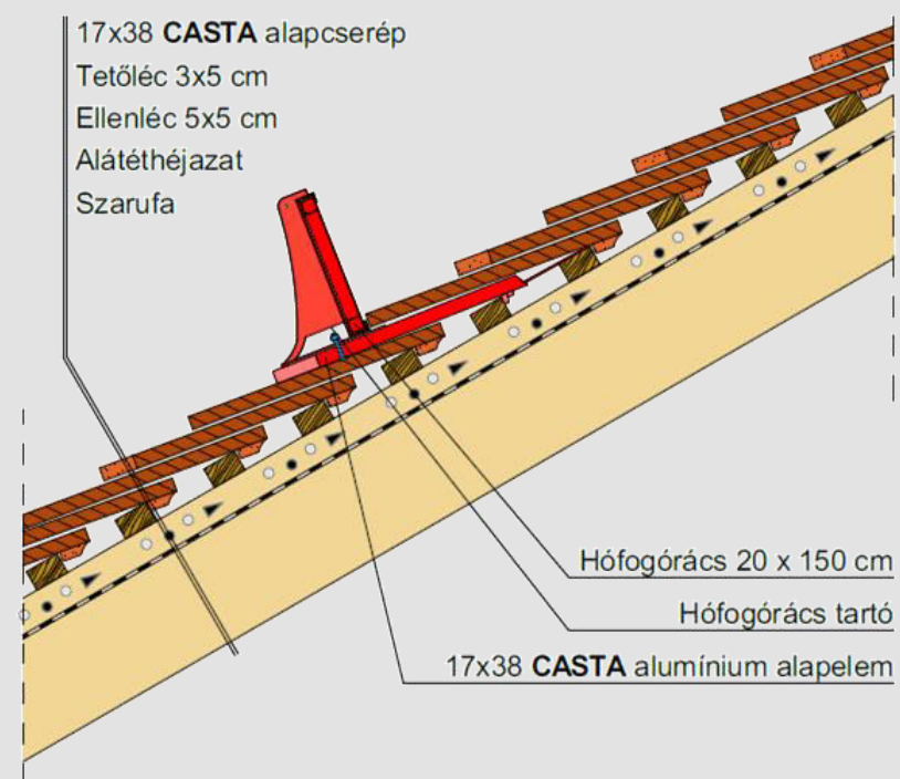
Hófogórács elhelyezése
