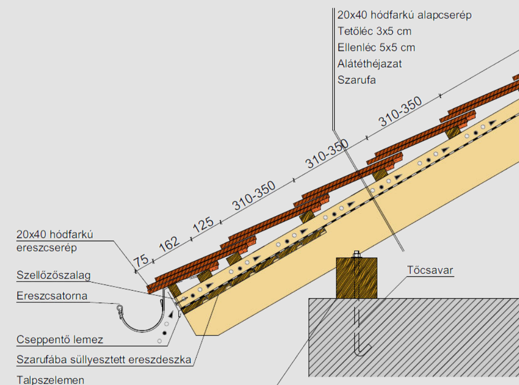
Koronafedésű ereszkialakítás
