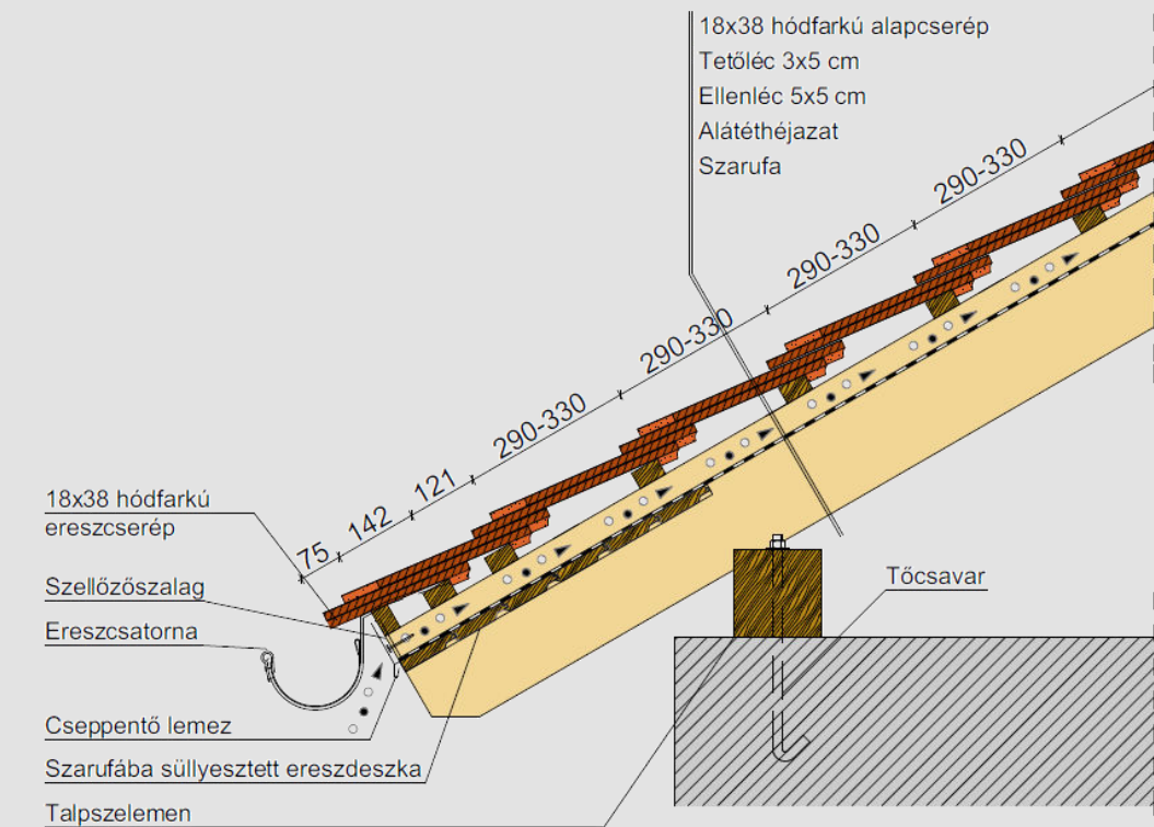
Koronafedésű ereszkialakítás
