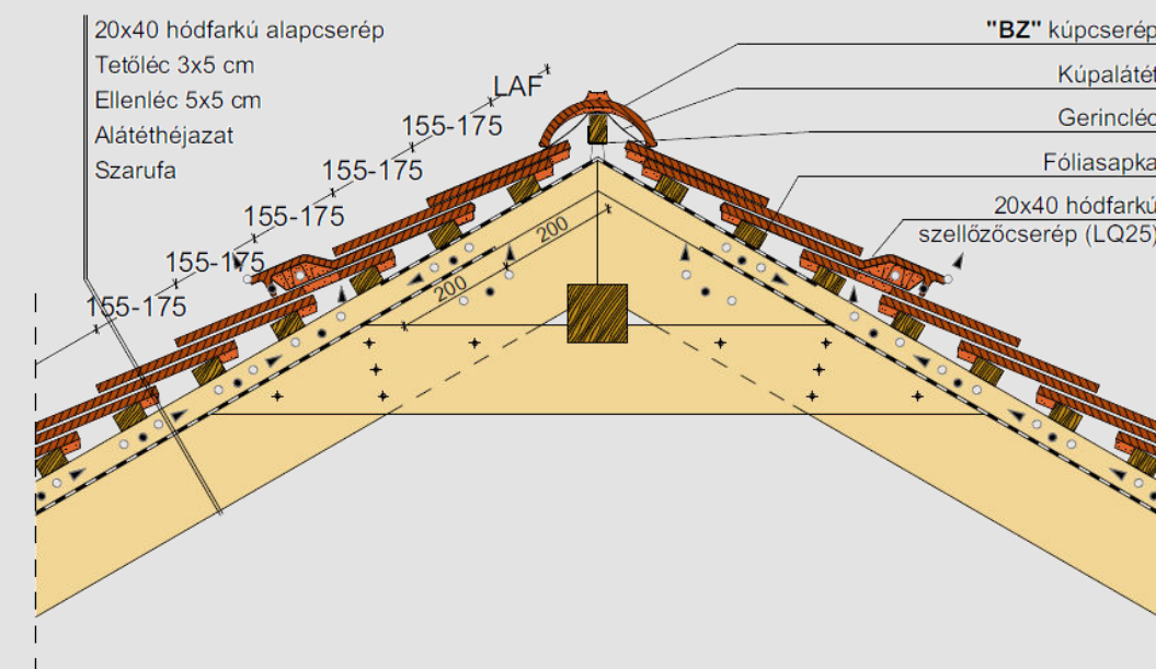
Gerinckialakítás, szellőzőcseréppel
