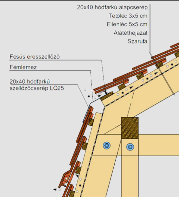
Negatív hajlásszögtörés kialakítás
