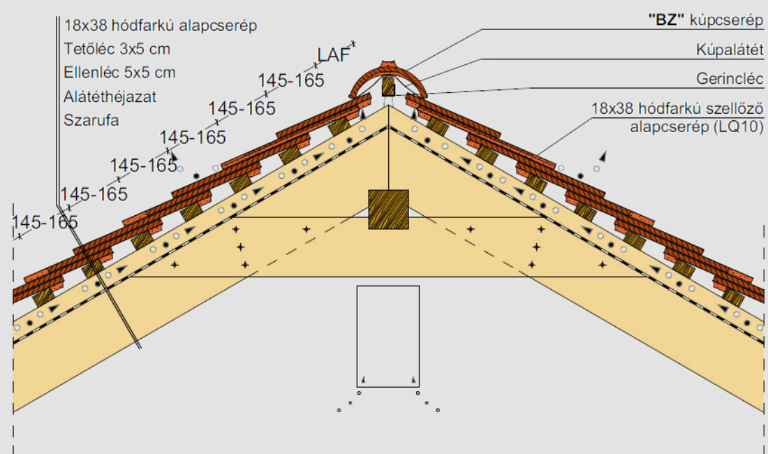
Gerinckialakítás, szellőző alapcseréppel
