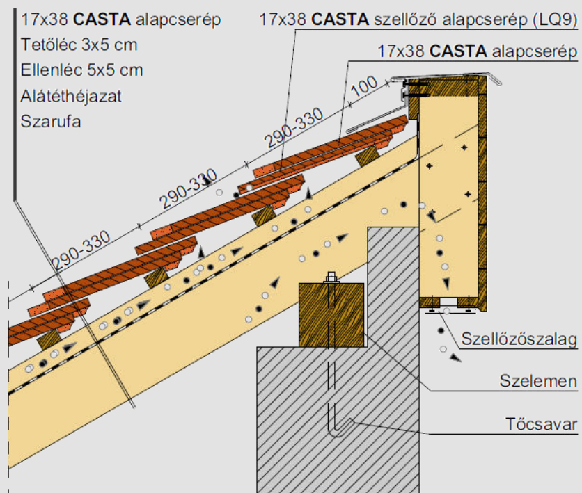
Koronafedésű félnyeregtető gerinc kialakítás
