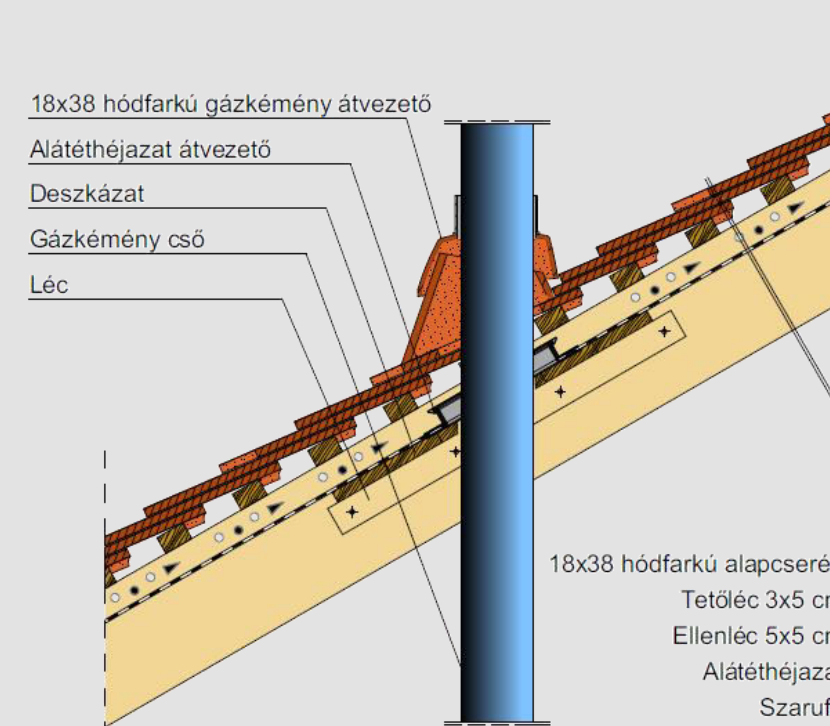
Kerámia gázkémény átvezető rendszer
