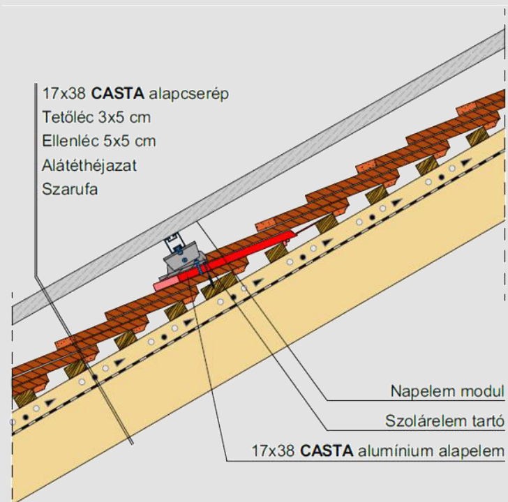
Alumínium szolárelem tartó elhelyezése
