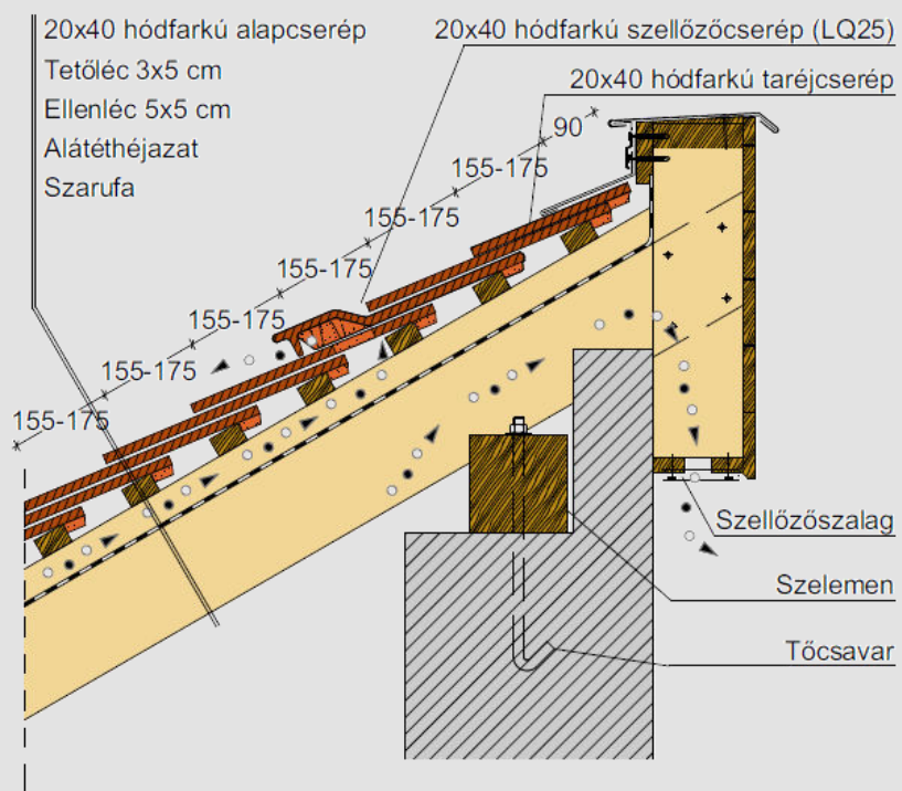
Félnyereg tető gerinc kialakítás
