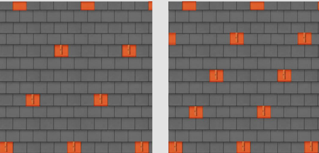
CREATON "Bécsi táska", kettősfedésben, 33,3 db/m 2 anyagigénnyel
