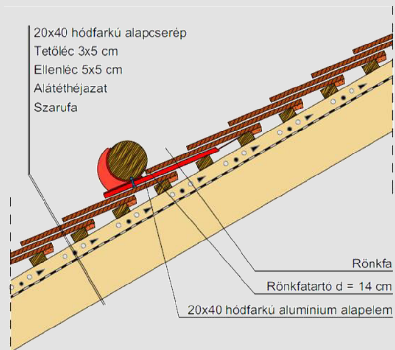
Rönkfartó elhelyezése
