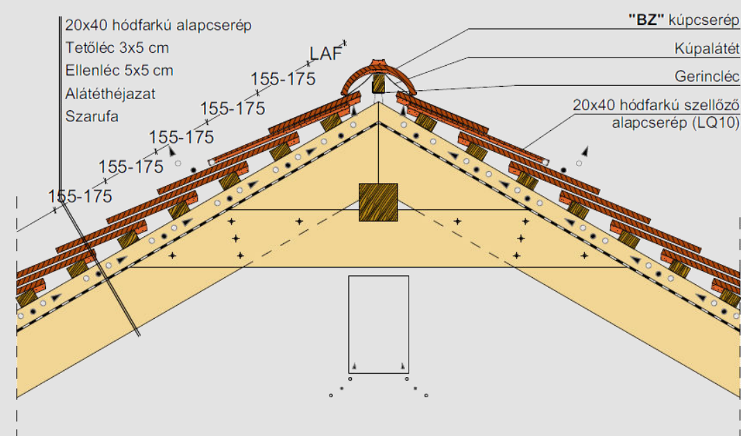
Gerinckialakítás, szellőző alapcseréppel
