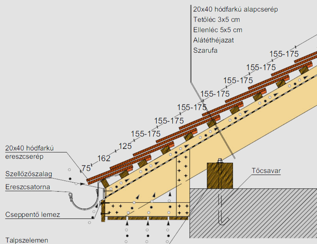
Dobozolt ereszkialakítás
