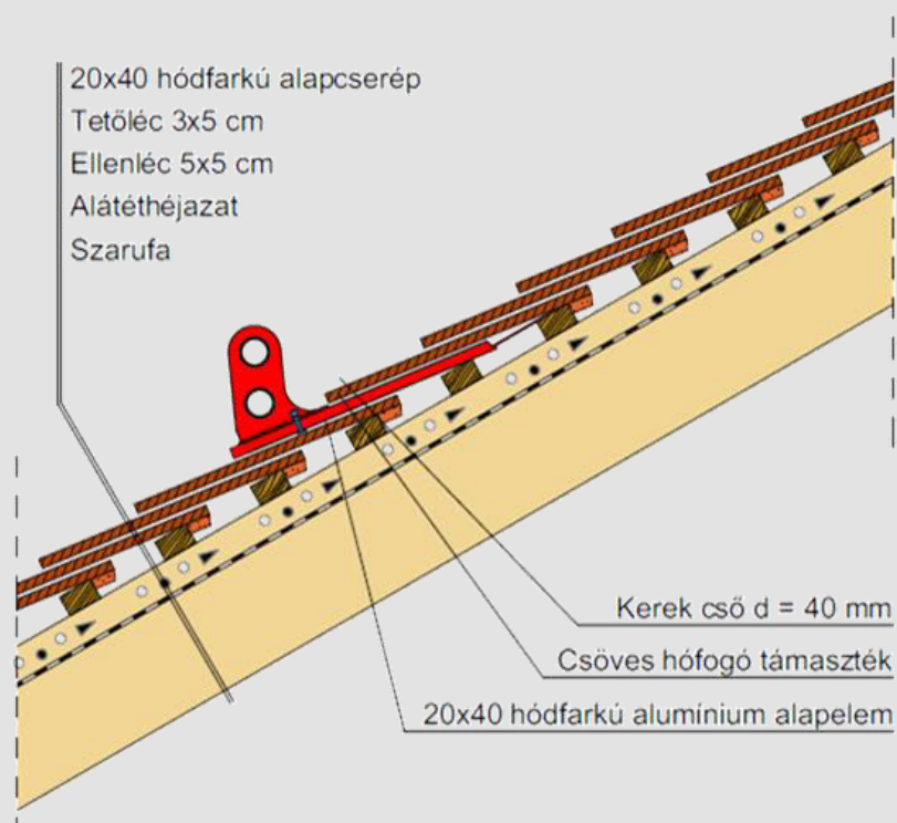
Hófogócső elhelyezése
