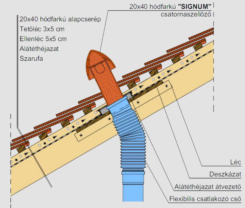
„SIGNUM“ kerámia csatornaszellőző átvezetés
