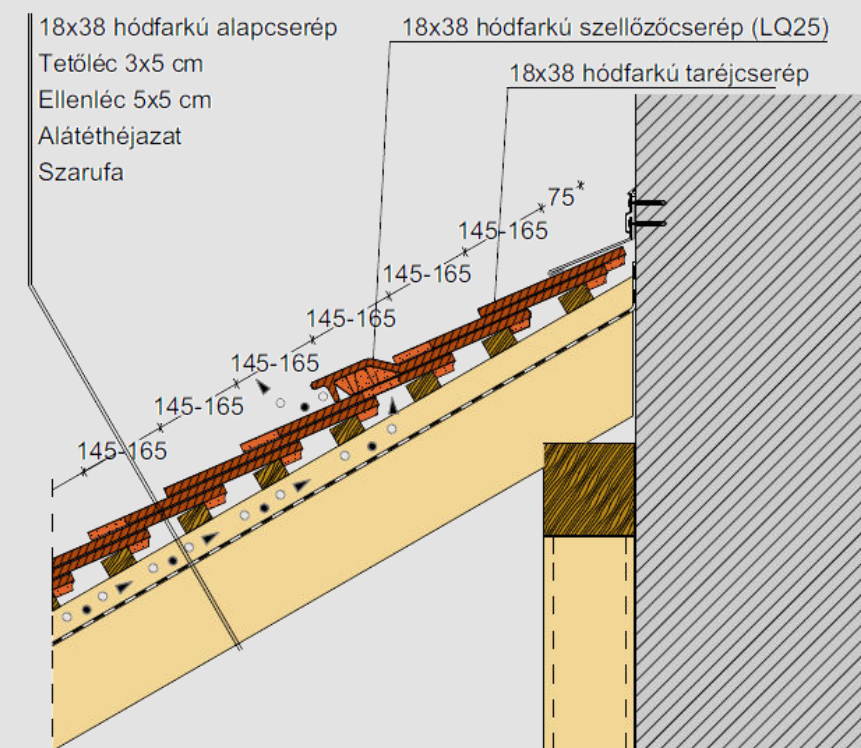
Falszegély kialakítás
