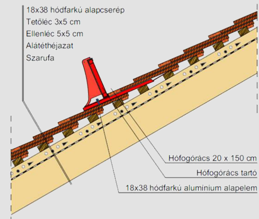
Hófogórács elhelyezése
