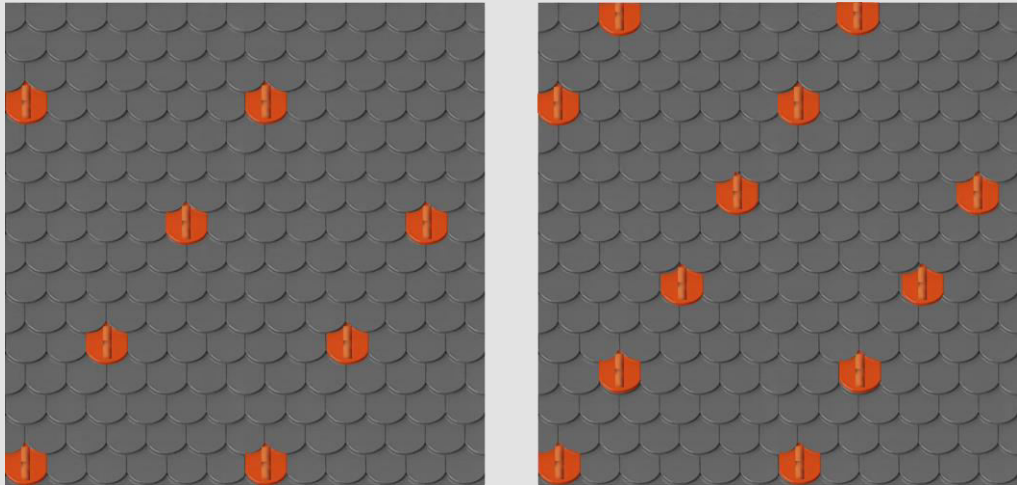
CREATON KLASSIK, kettősfedésben 37,0 db/m 2 anyagigénnyel
